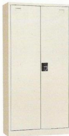
CY-032 掩门柜 Two Doors 尺寸Size: W800•D400•H1800mm 毛重G. Weight: 41kgs 包装体积Packing Volume: 0.131cbm
